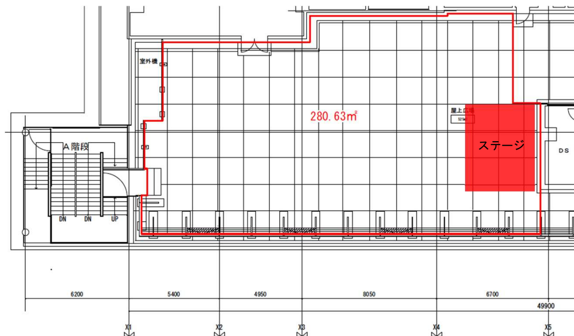
<平面図>
